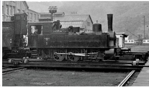
Als letzte Werklok im Einsatz 1958 bei der ME
